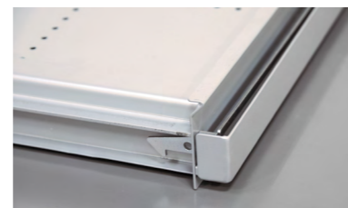
圖 1. 驅動板安全勾設計
